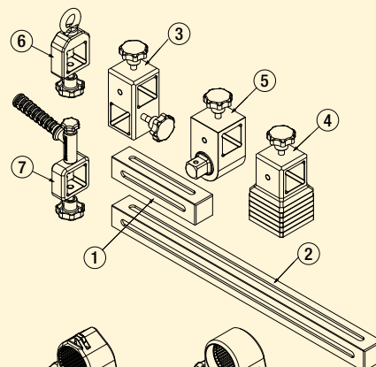
TWRAKSL * Adaptereinheit für Drehmoment-schlüssel der RSL-Serie
