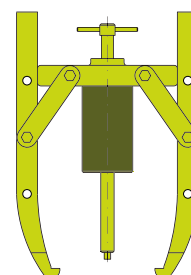
Extractor de garras FX - FV
