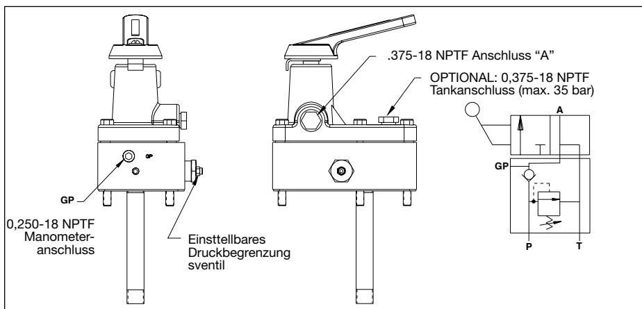
Abbildung 2, VM22, Pumpe montiert
