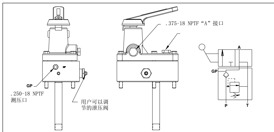
图 2, VM22, 安装的泵
