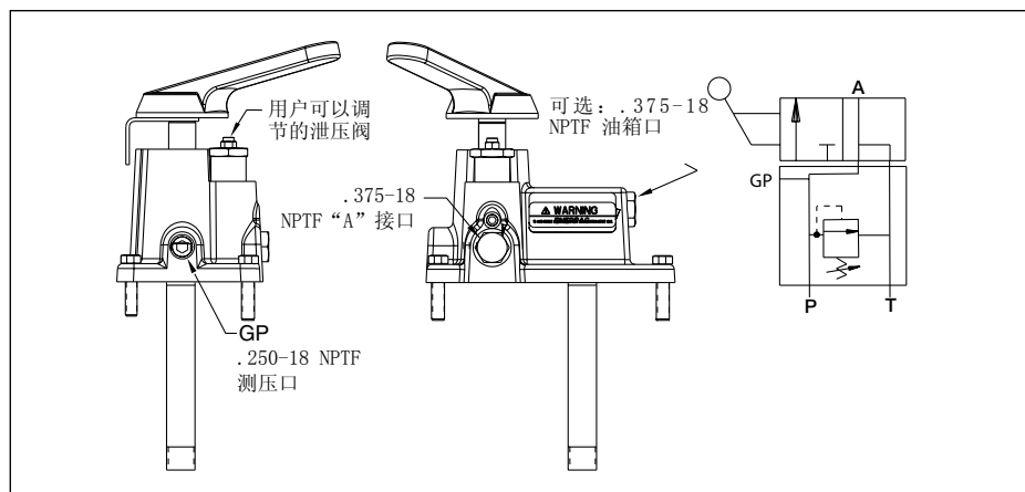
图1, VM32, 安装的泵
