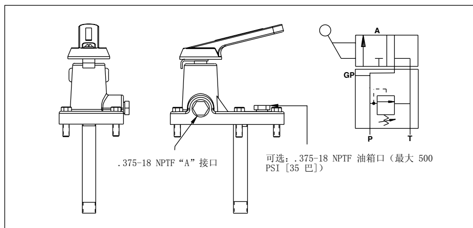
图 3, VM2, 安装的泵
