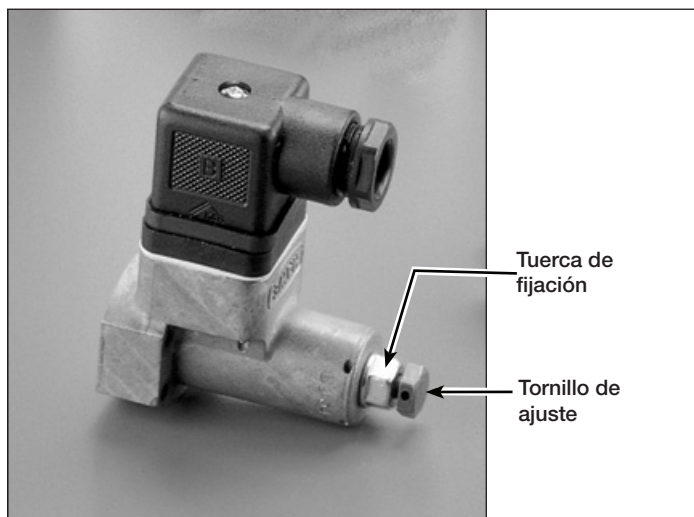
Figura 10 Presostato
