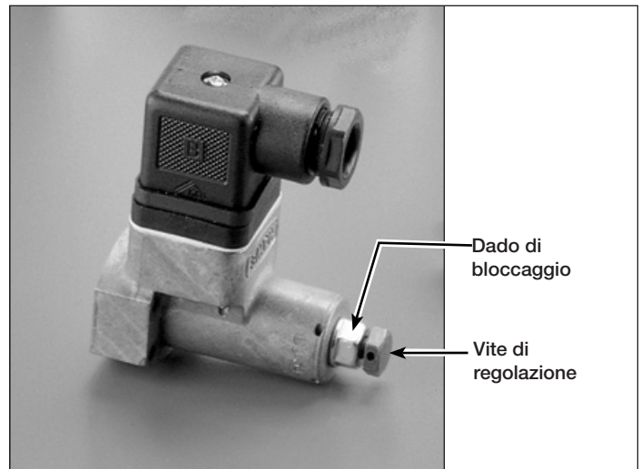
Figura 10, Pressostato
