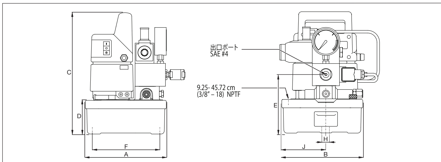
図1 外寸
