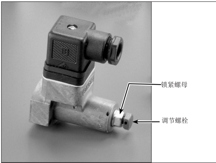
图 10, 压力开关
