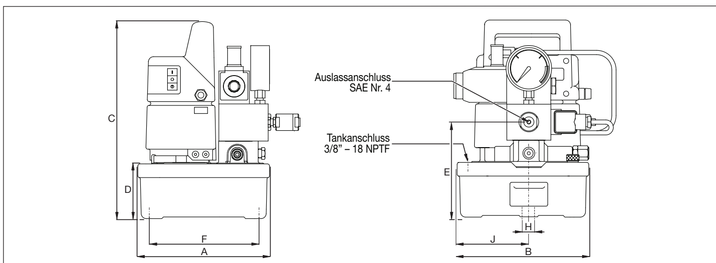
Abb. 1, Außenabmessungen
