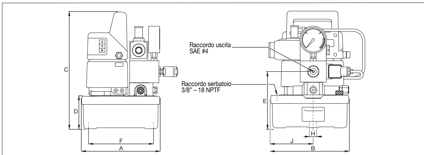
Figura 1, Dimensioni Esterne
