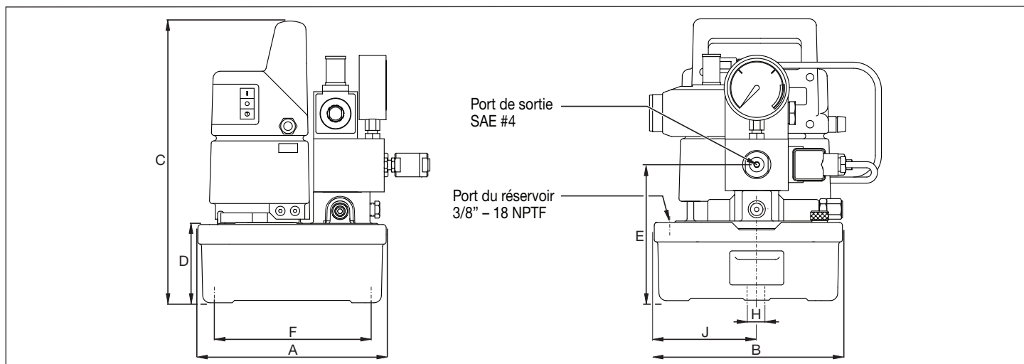
Figure 1, Dimensions extérieures
