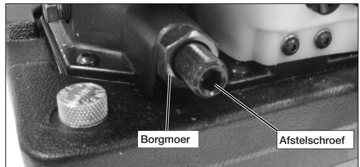
Figuur 9, Externe ontlastklep (inbuskopschroef verwijderd)
