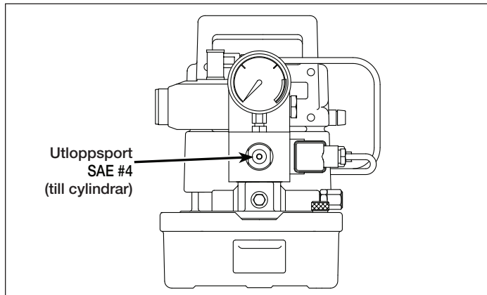
Figur 3, Reglerventilen utloppsport
