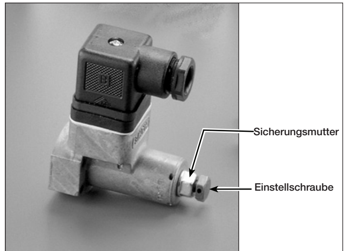
Abb. 10, Druckschalter
