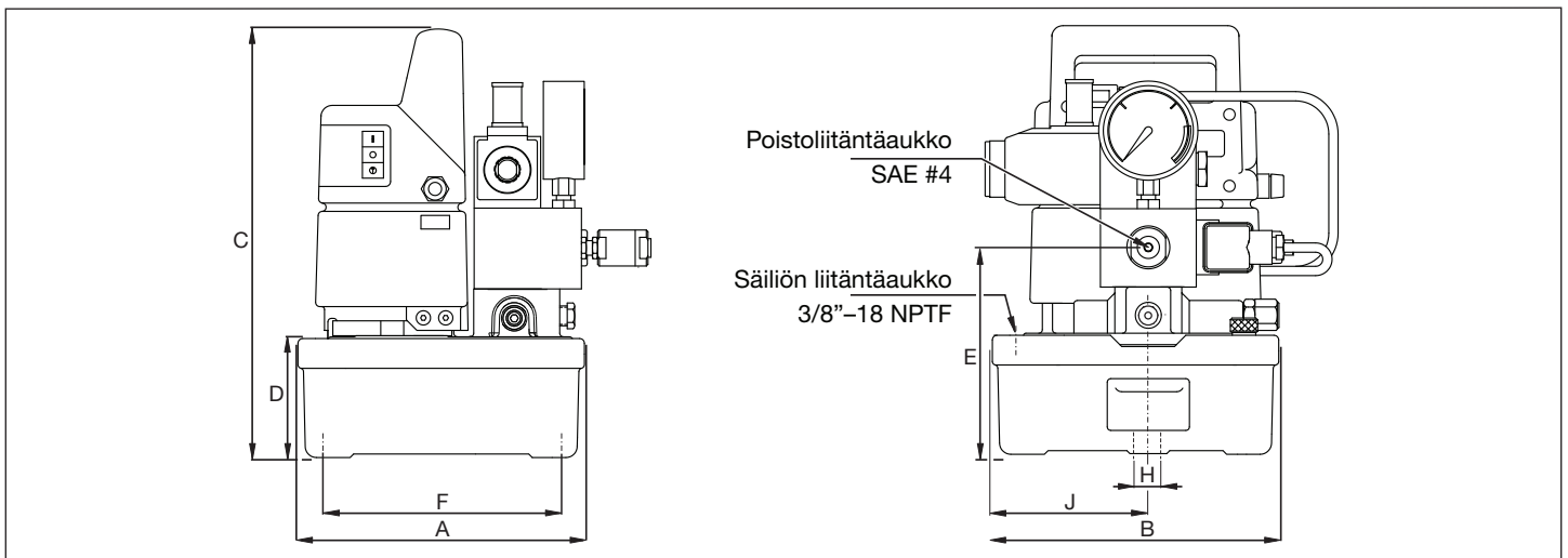
Kuva 1, Ulkomitat
