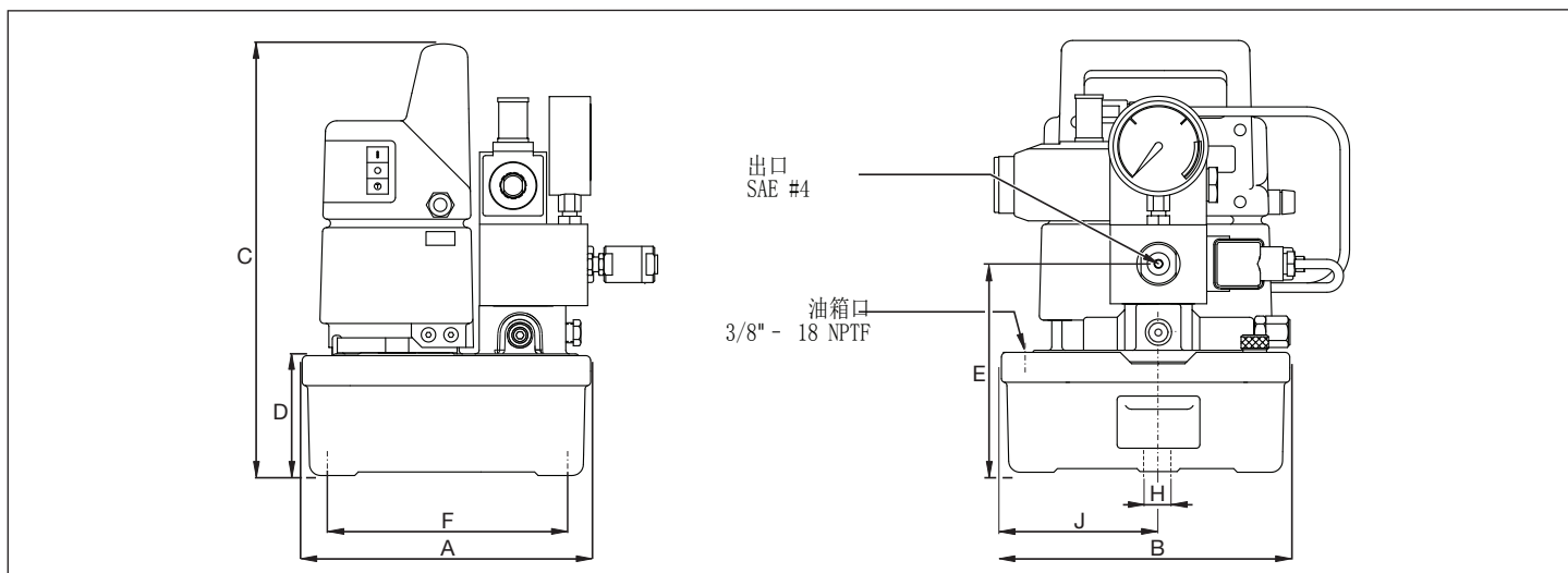
图 1，外部尺寸
