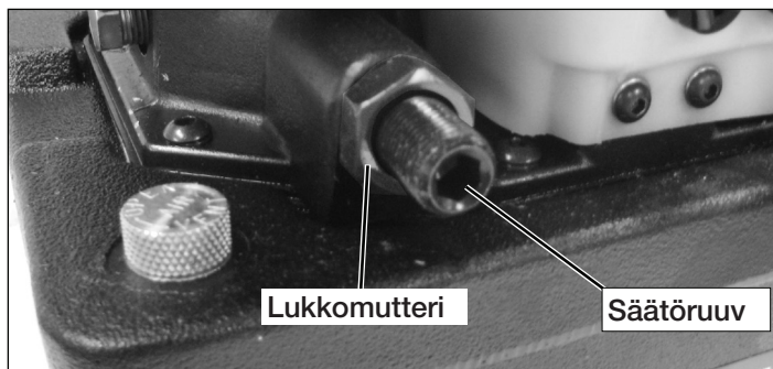
Kuva 9, Ulkoinen varoventtiili (kuusiokolo irrotettuna)
