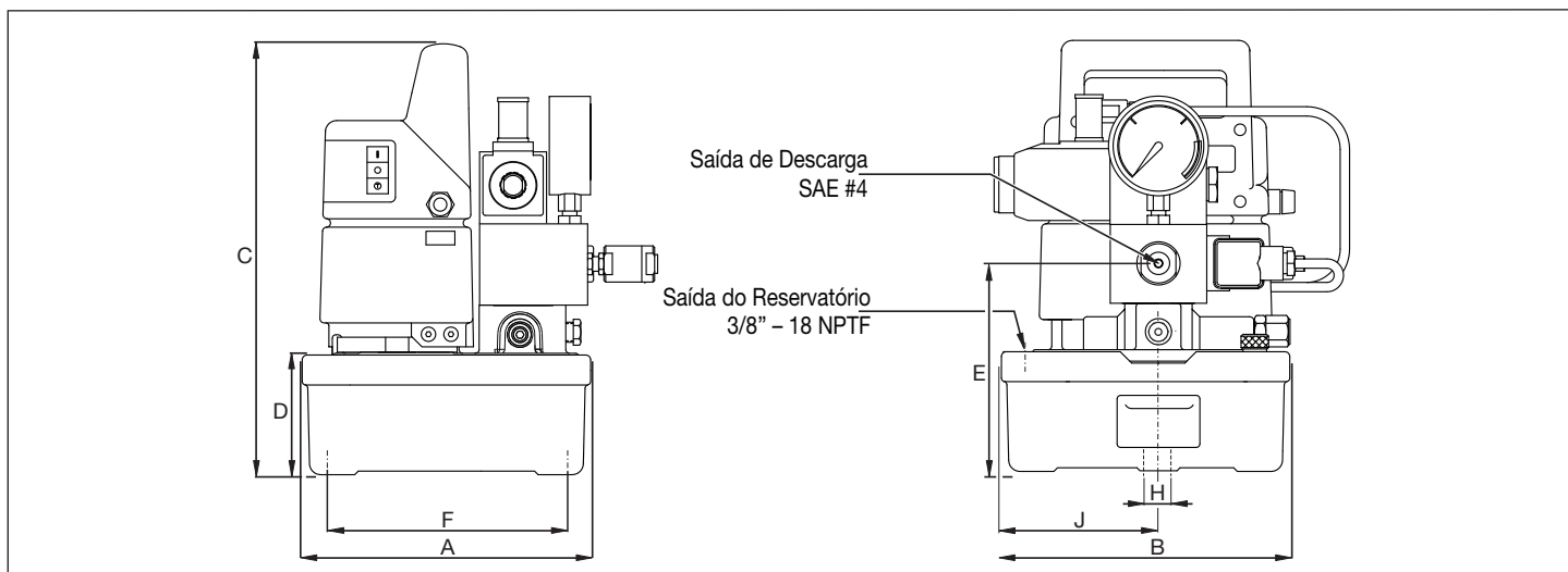
Figura 1, Dimensões Externas
