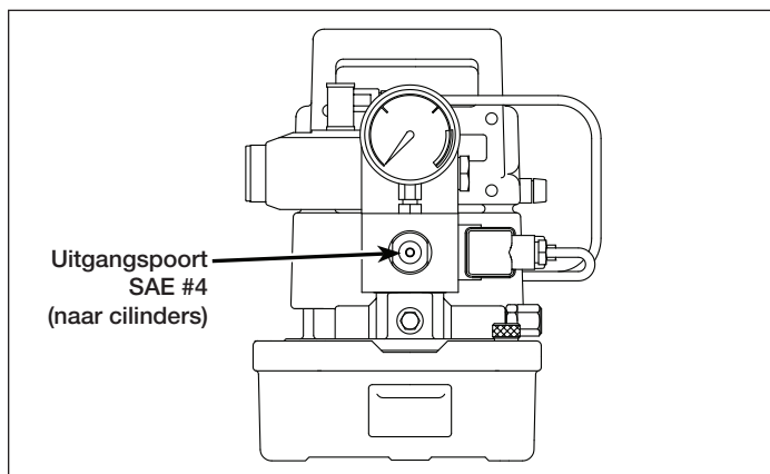
Figuur 3, Regelklep uitgangspoort
