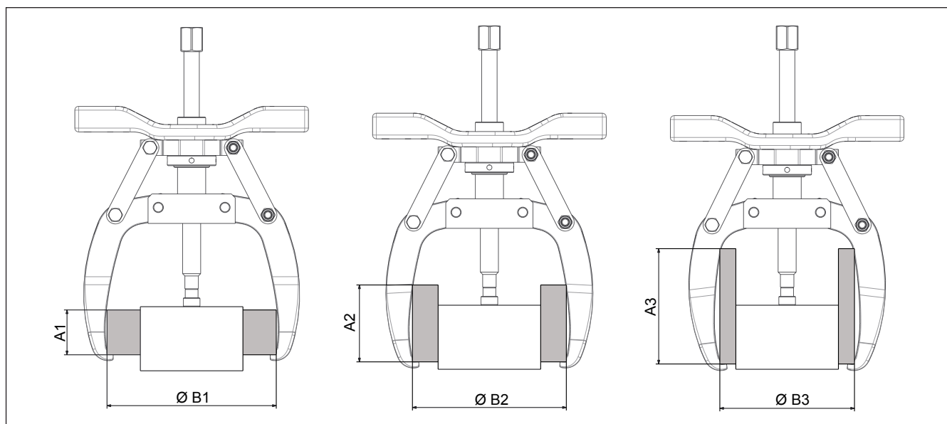
図6: プーラーの最大リーチとスプレッド
