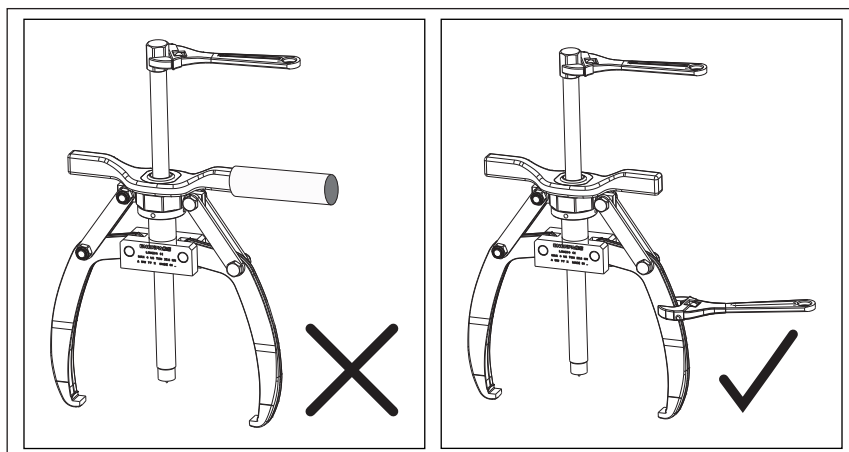
図5: プーラーの保持推奨事項
