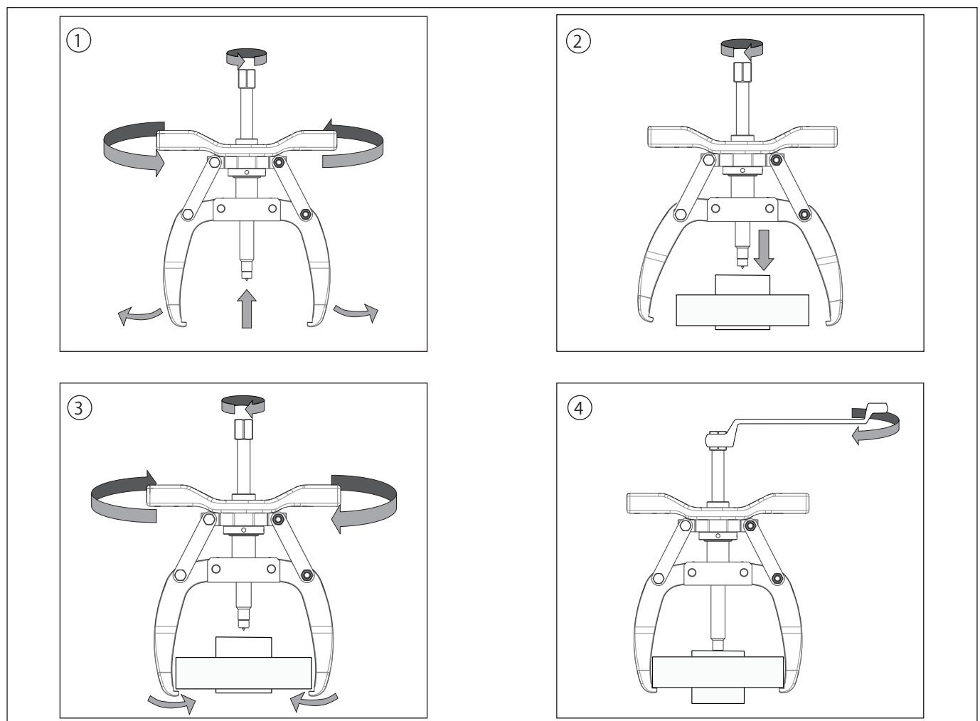
図3: プーラーの設置手順
