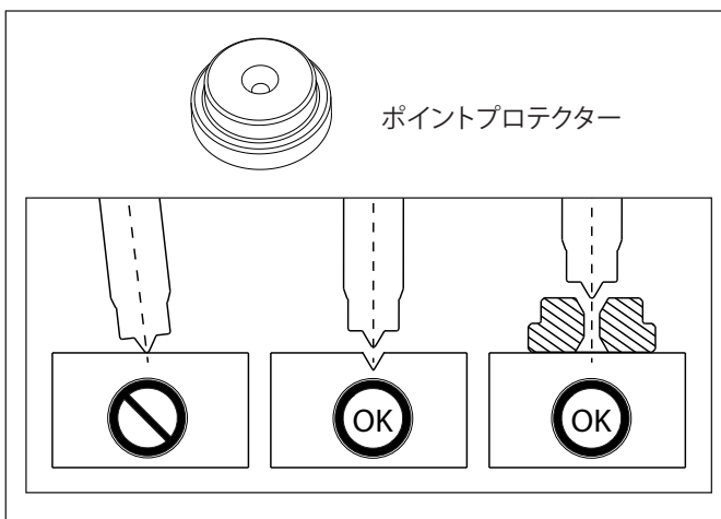
図2: ポイントプロテクター
