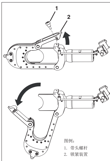
图 4，打开切割头
