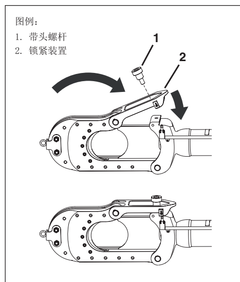
图 5，关闭切割头
