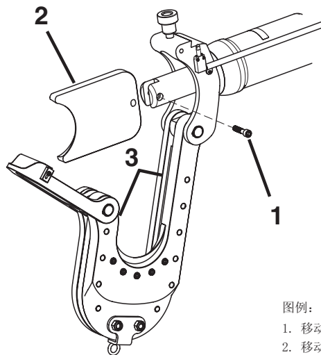
图 12，移动刀片更换
