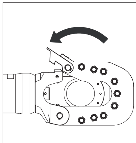
図6：カuttingヘッドが閉じた状態
