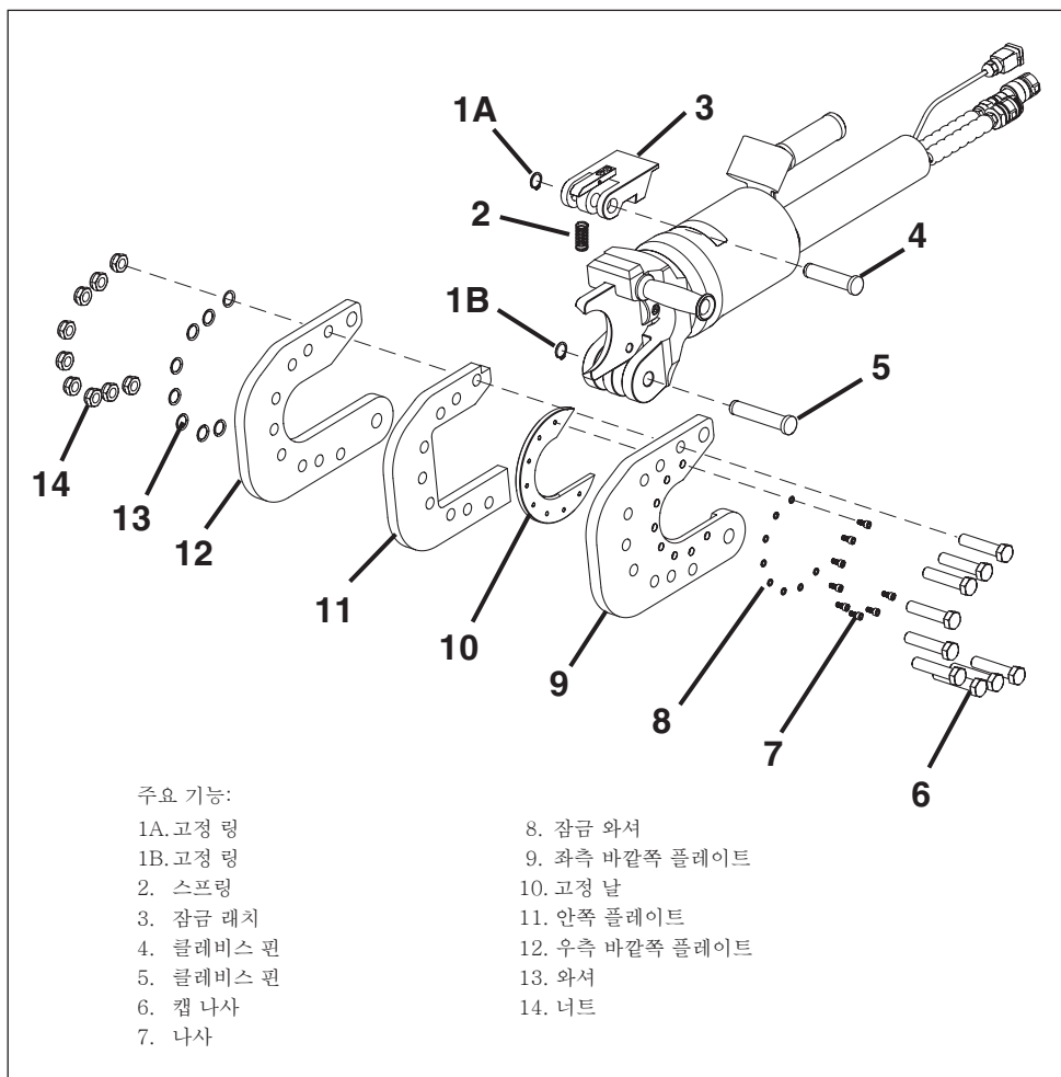
그림 12. 고정 날 교체(모델 EWCH90 표시됨, EWCH140도 유사함)
