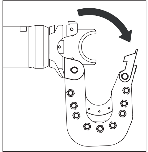
그림 5. 커팅 헤드 열기
