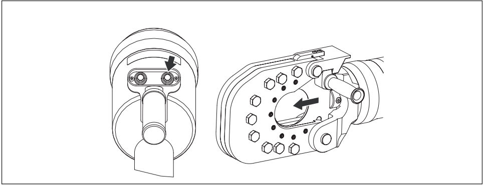
그림 10. 작동 - 전진/절단
