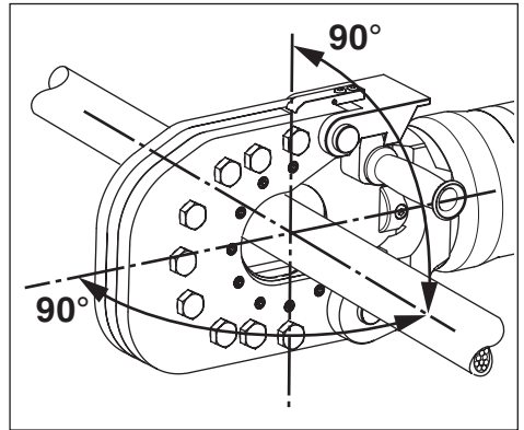
그림 9. 커팅 헤드의 재료 배치
