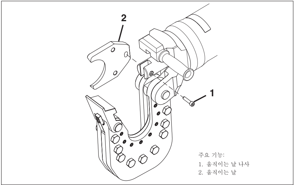
그림 13, 움직이는 날 교체(모델 EWCH90 표시됨, EWCH140도 유사함)
