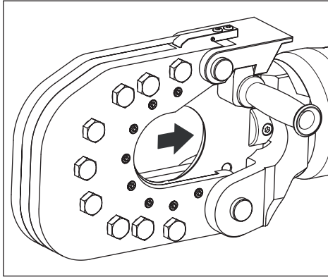
그림 8. 홈 위치의 피스톤과 날 (완전히 후진한 상태)
