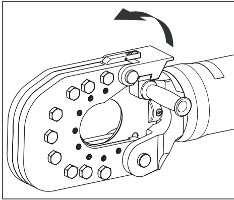
그림 4. 잠금 래치
