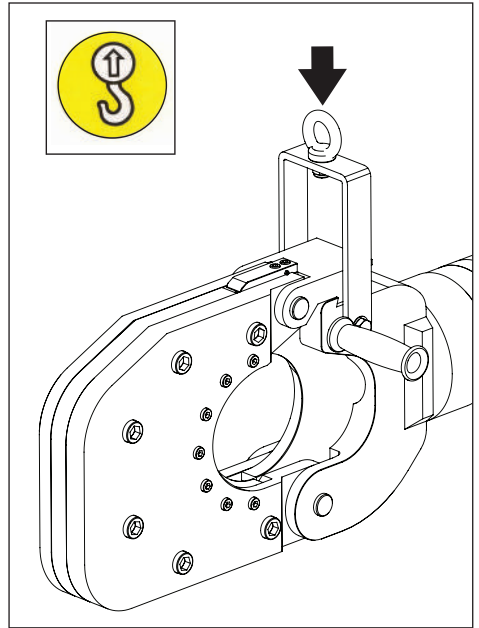
그림 7, 절단기 리프팅 위치
