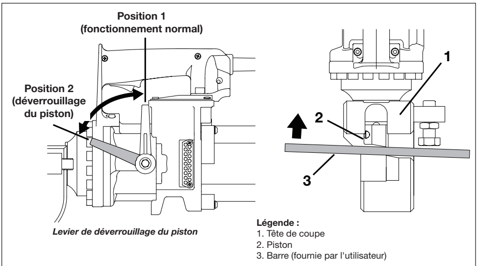
Image 11, Procédure de rétraction manuelle du piston
