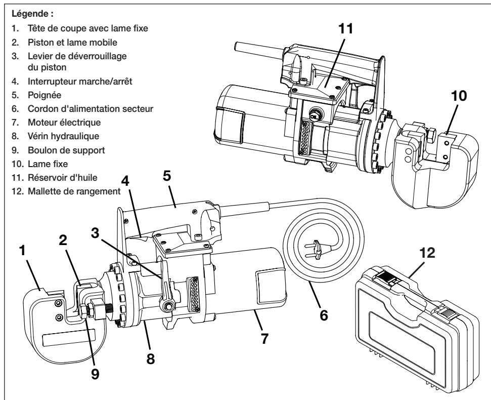
Image 1- Caractéristiques et composants
