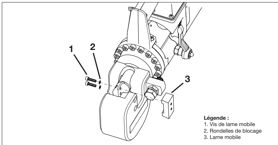
Image 10, Remplacement de la lame mobile
