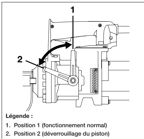
Image 5, Levier de déverrouillage du piston
