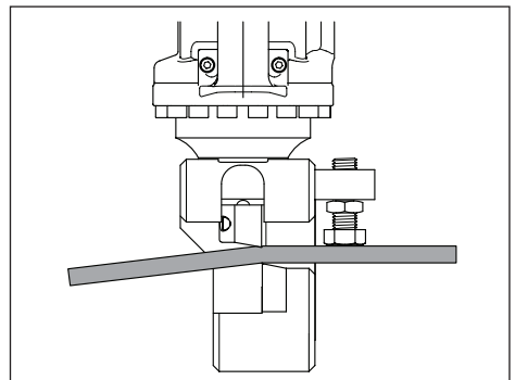
Image 7, Objet en cours de coupe (vue du dessus)
