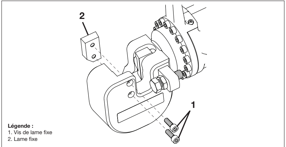
Image 9, Remplacement de la lame fixe
