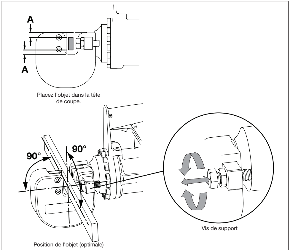
Image 6, Positionnement de l'objet dans la tête de coupe
