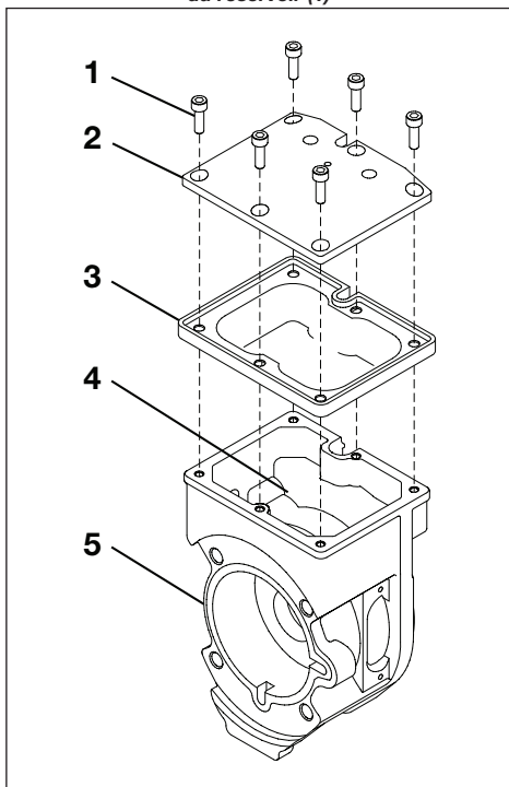
Image 8E, vis (1), couvercle de membrane (2), membrane (3), ouverture de membrane (4) et réservoir (5)
