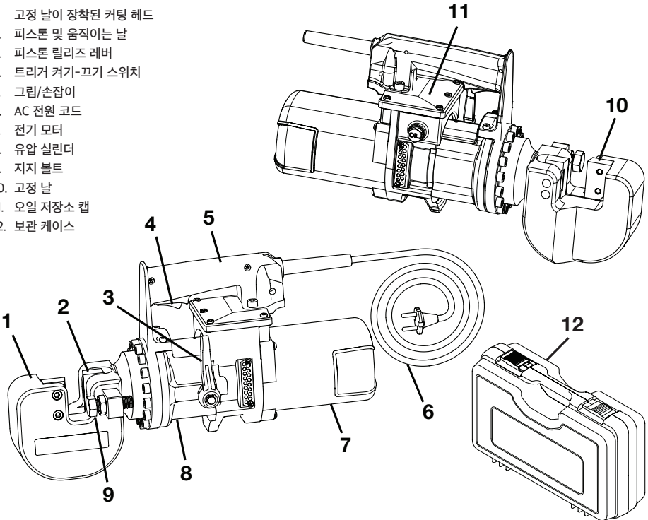
그림 1. 기능 및 구성품
