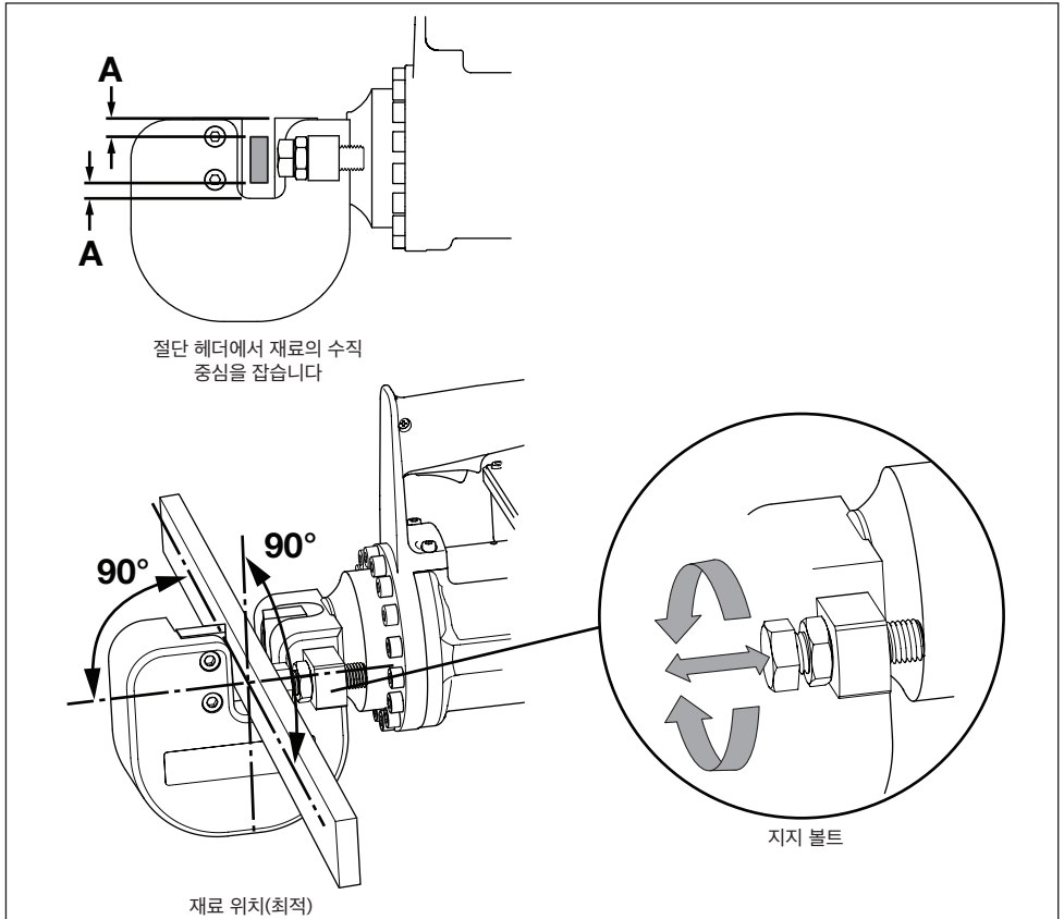
그림 6. 커팅 헤드 내 재료 위치
