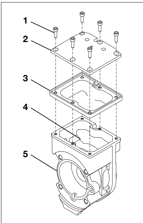
그림 8E, 나사 (1), 다이어프램 커버 (2), 다이어프램 (3), 다이어프램 입구 (4) 저장소 (5)
