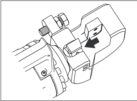
그림 4, 피스톤과 블레이드가 완전히 후진한 ("흡") 위치
