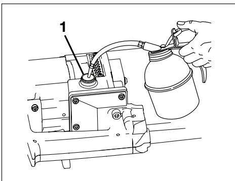
그림 8D, 저장소 보충 구멍에 오일 추가 (1)
