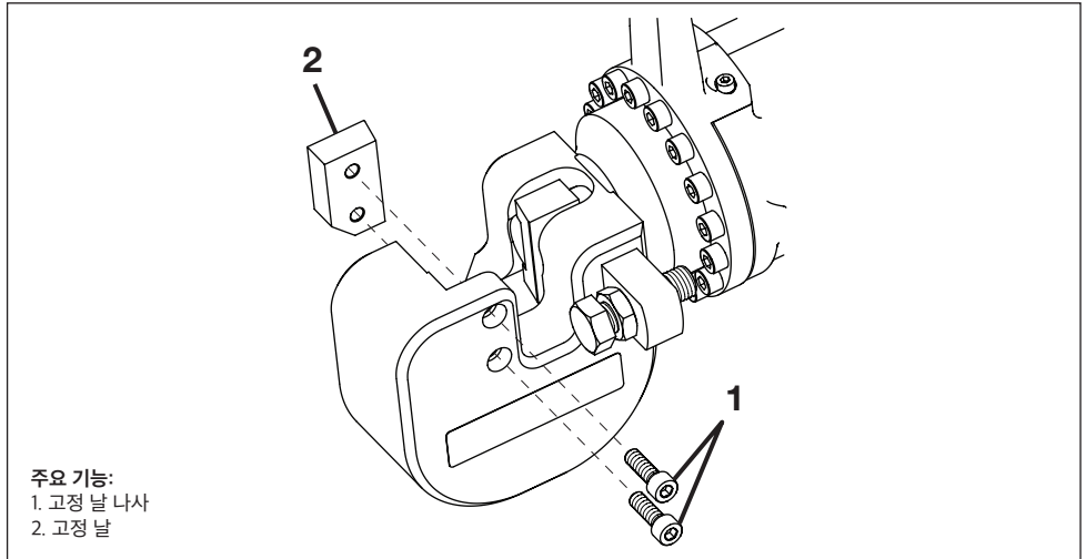
그림 9, 고정 날 교체
