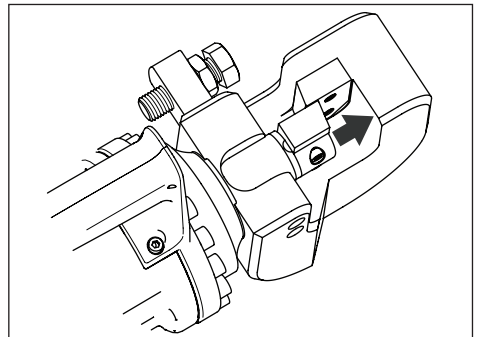
Figuur 3. Plunjer en snijmes volledig uitgelopen
