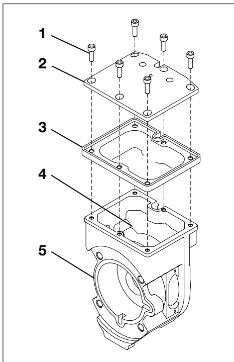
Figuur 8E. Schroeven (1), afsluiting membraan (2), membraan, (3), opening membraan (4) en reservoir (5)
