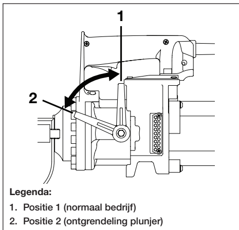
Figuur 5. Blokkeerhandgreep
