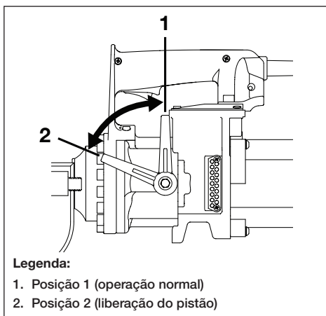
Figura 5, alavanca de liberação do pistão
