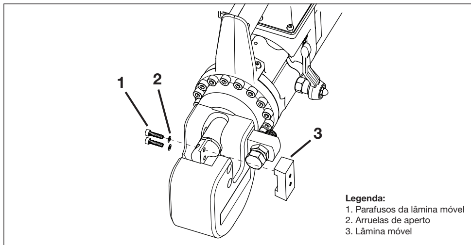
Figura 10, troca da lâmina móvel
