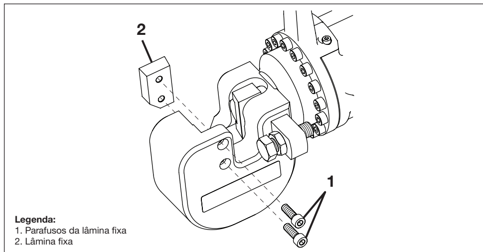
Figura 9, troca da lâmina fixa
