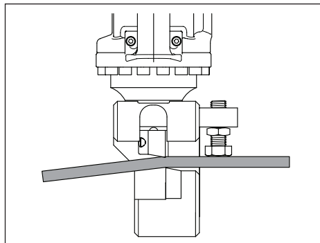
Figura 7, material sendo cortado (típico - vista de cima)
