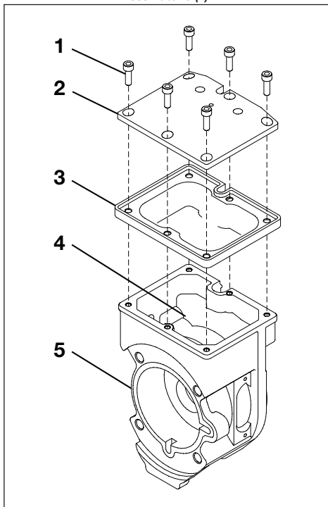
Figura 8E, parafusos (1), tampa do diafragma (2), diafragma (3), abertura do diafragma (4) e reservatório (5)
