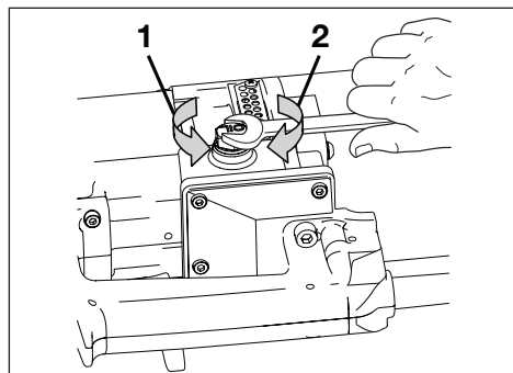
Figura 8C, tampa do reservatório de óleo - solto (1) e apertado (2)
