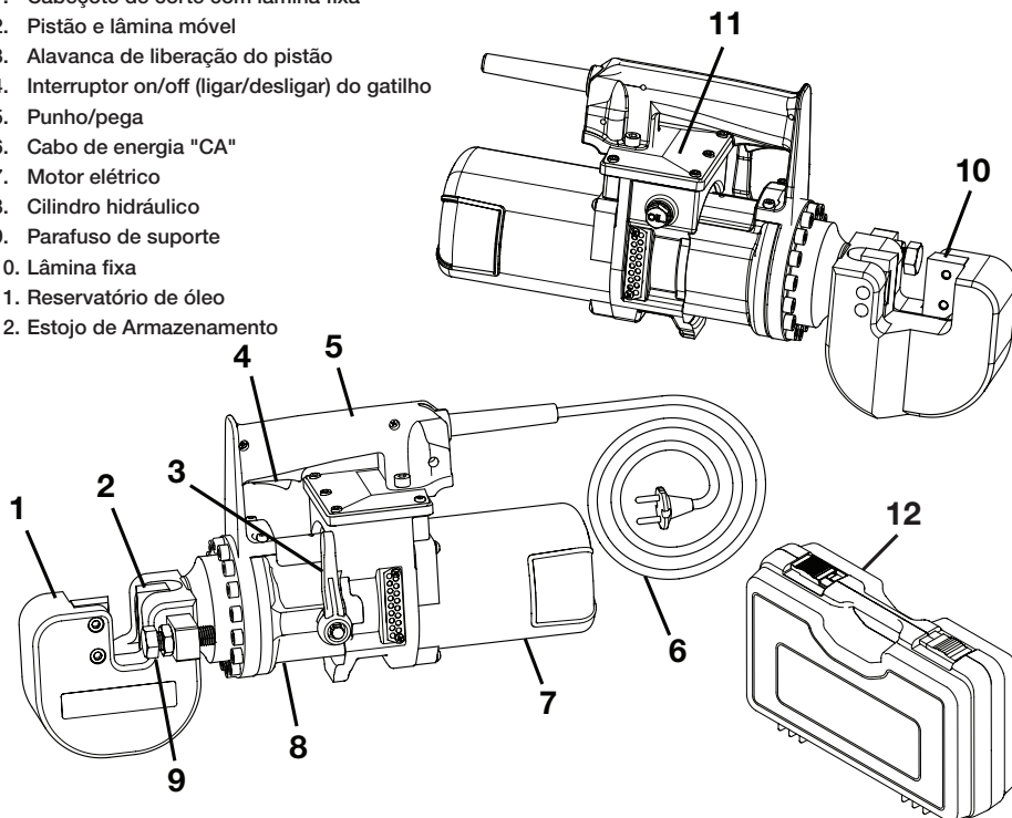
Figura 1, características e componentes
