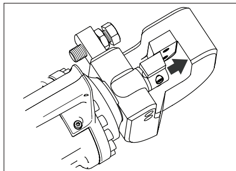
Figura 3, pistão e lâmina totalmente avançados
