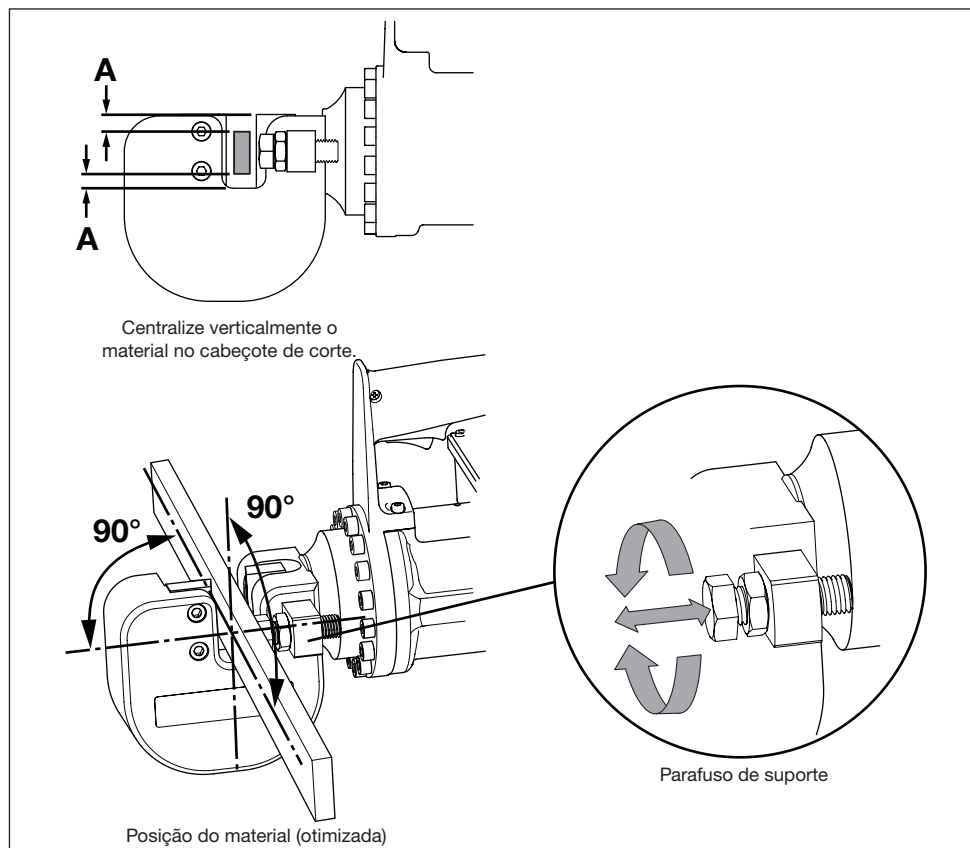
Figura 6, posicionamento do material no cabeçote de corte
