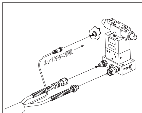
図3: ポンプ部の油圧接続部および電気接続部
