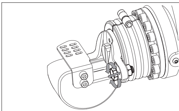
図8:支持ボルトの調整
