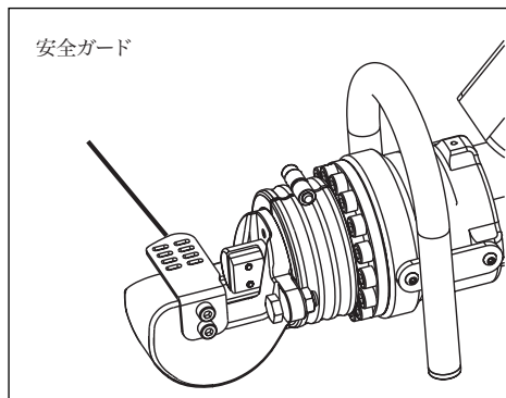
図4: 安全ガード
