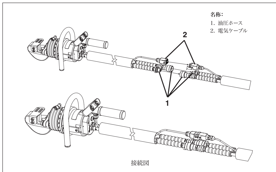
図2:カッター部の油圧接続部および電気接続部(一般的)
