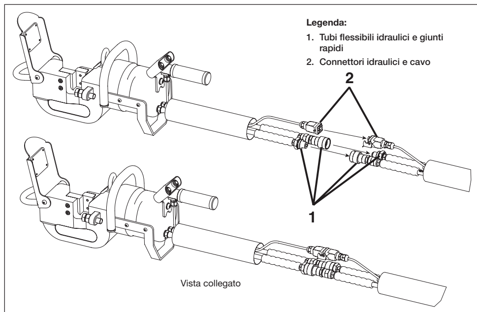
Figura 2, Collegamenti idraulici ed elettrici del tagliabarre (configurazione tipica)
