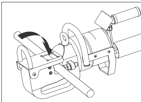
Figura 6, Chiusura della protezione
