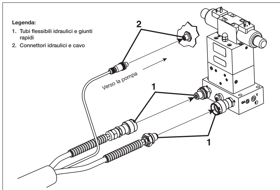
Figura 3, Collegamenti idraulici ed elettrici della pompa
