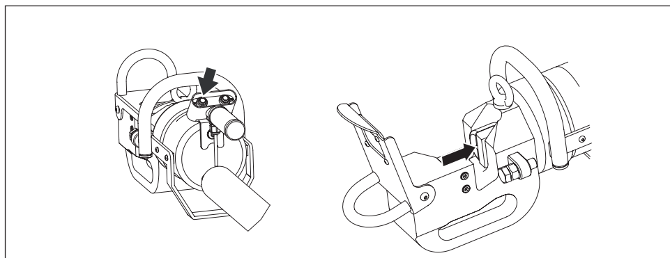
Figura 12, Funzionamento - Retrazione
