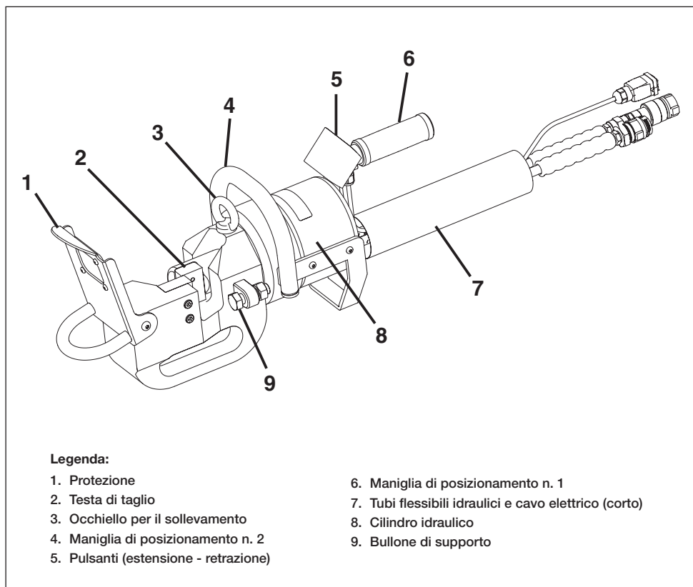
Figura 1, Caratteristiche e componenti
