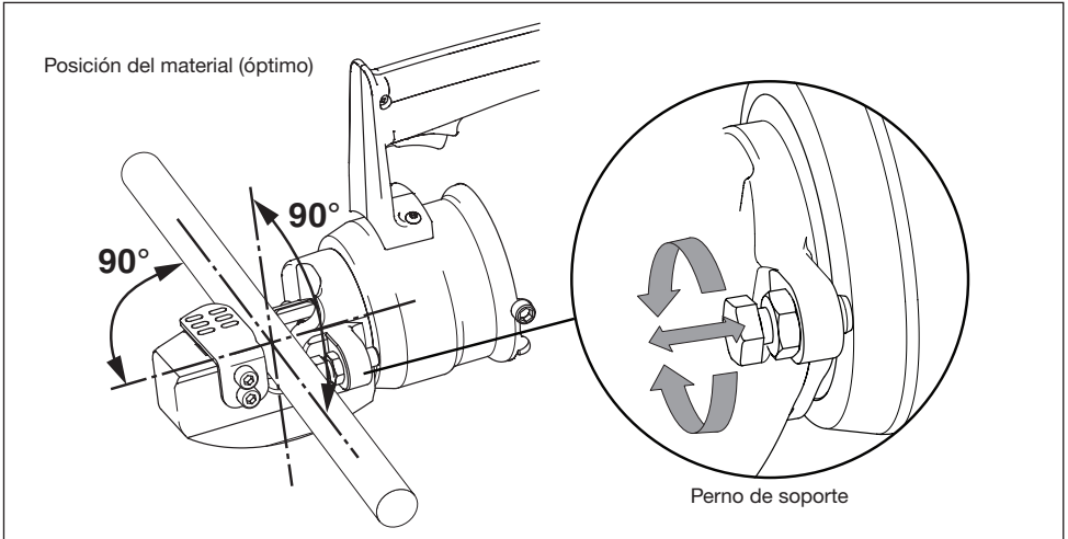
Figura 6, Colocar el material en el cabezal de corte
