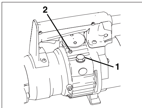
Figura 8A, Tapón del depósito de aceite (1) y el tornillo de purga (2)
