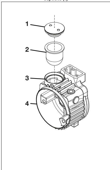
Figura 8E, Tapa de diafragma (1), Diafragma (2), Abertura de diafragma (3) y Depósito de aceite (4)
