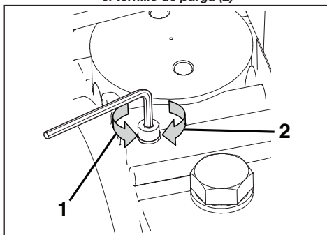
Figura 8B, Tornillo de purga - Apretar (1) y aflojar (2)
