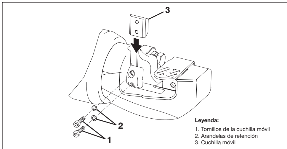
Figura 10, Sustitución de cuchilla móvil
