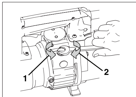
Figura 8C, Tapón del depósito de aceite - Aflojar (1) y apretar (2)
