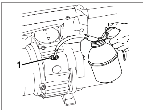
Figura 8D, Añadir aceite en el agujero de llenado del depósito (1)
