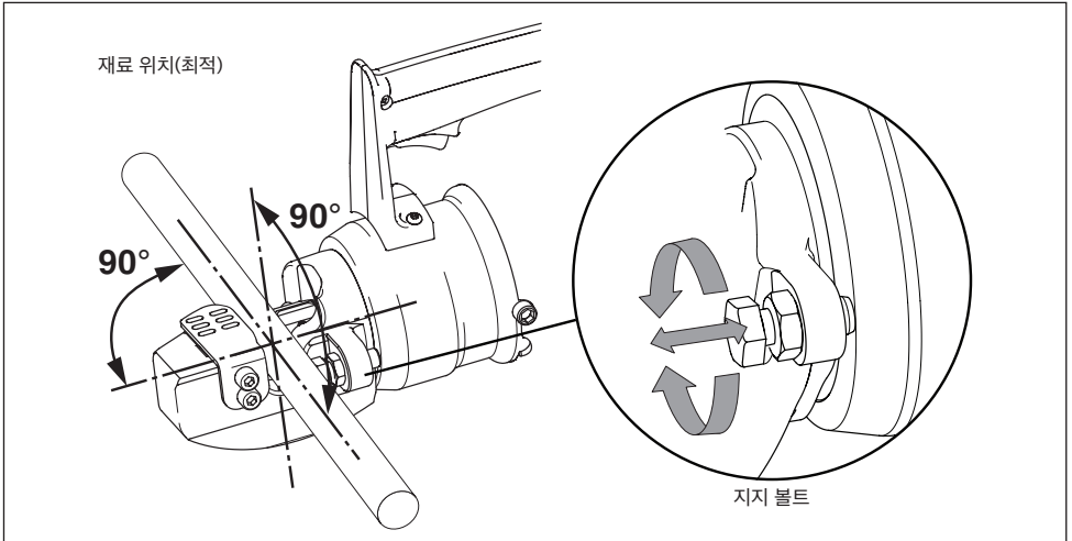
그림 6. 커팅 헤드 내 재료 위치
