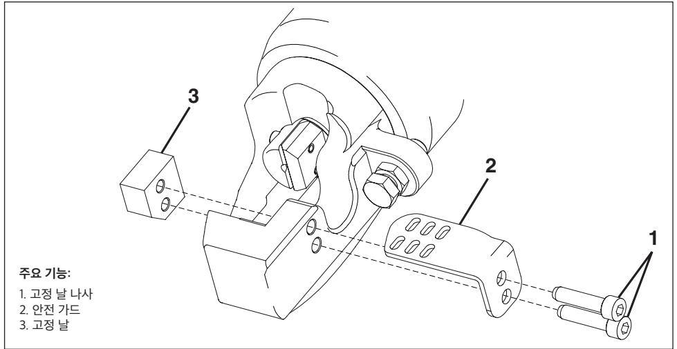
그림 9, 고정 날 교체
