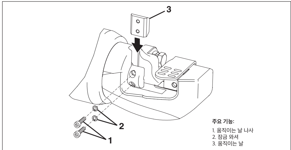
그림 10. 가동 날 교체
