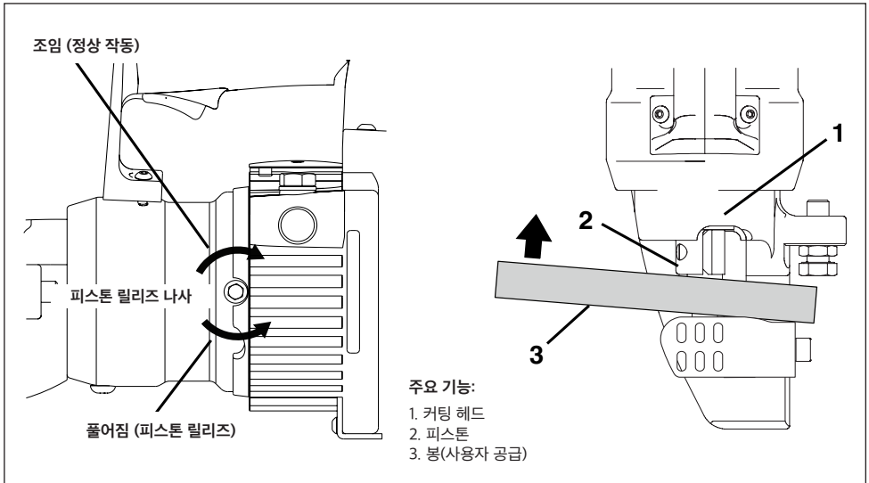
그림 11, 피스톤 수동 후진 절차
