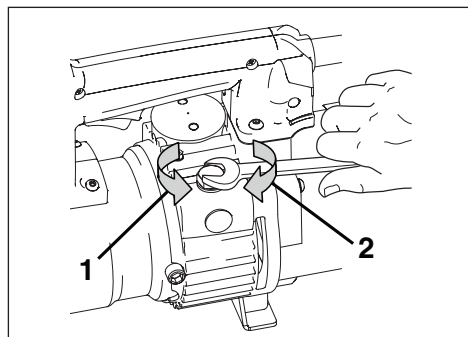
그림 8C, 오일 저장소 캡 - 풀림 (1) 및 조임 (2)
