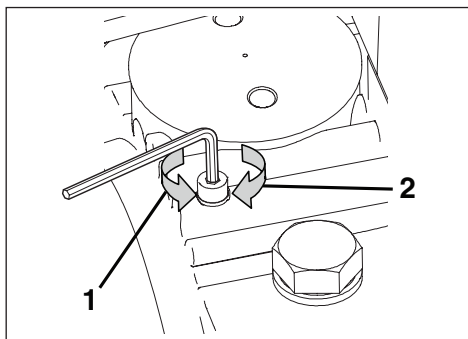
그림 8B, 환기구 나사 - 풀림 (1) 및 조임 (2)
