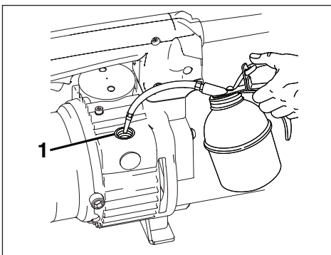
그림 8D, 저장소 보충 구멍에 오일 추가 (1)
