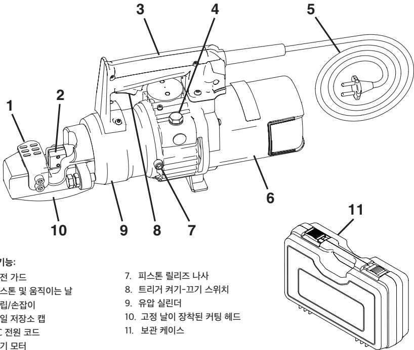
그림 1. 기능 및 구성품
