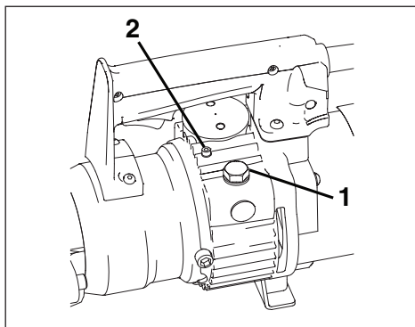
Figuur 8A. Dop van oliereservoir (1) en ontluchtingsschroef (2)
