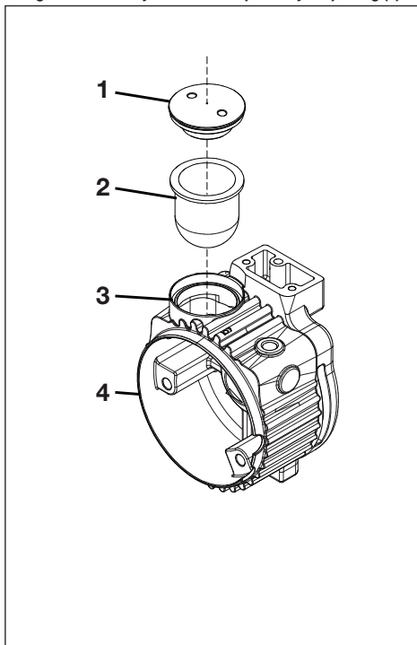
Figuur 8E. Afsluiting membraan (1), membraan, (2), opening membraan (3) en oliereservoir (4)
