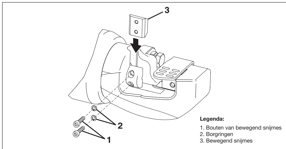
Figuur 10. Bewegend snijmes vervangen
