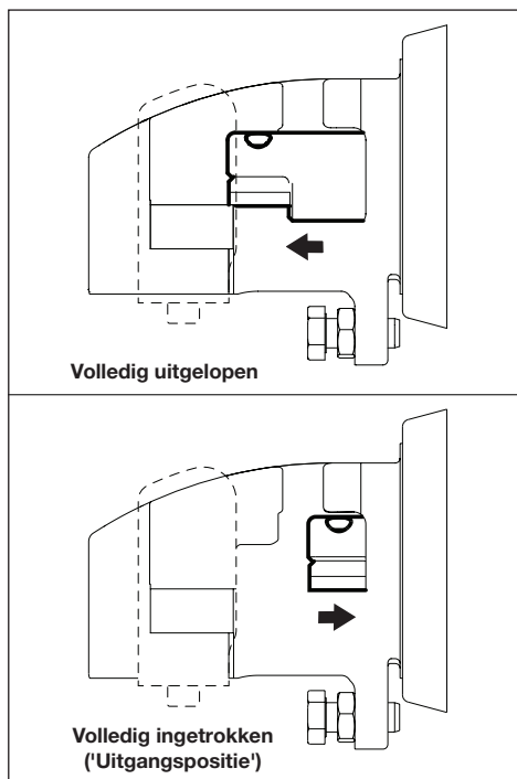
Figuur 3. Plunjerstanden (bovenaanzicht)
