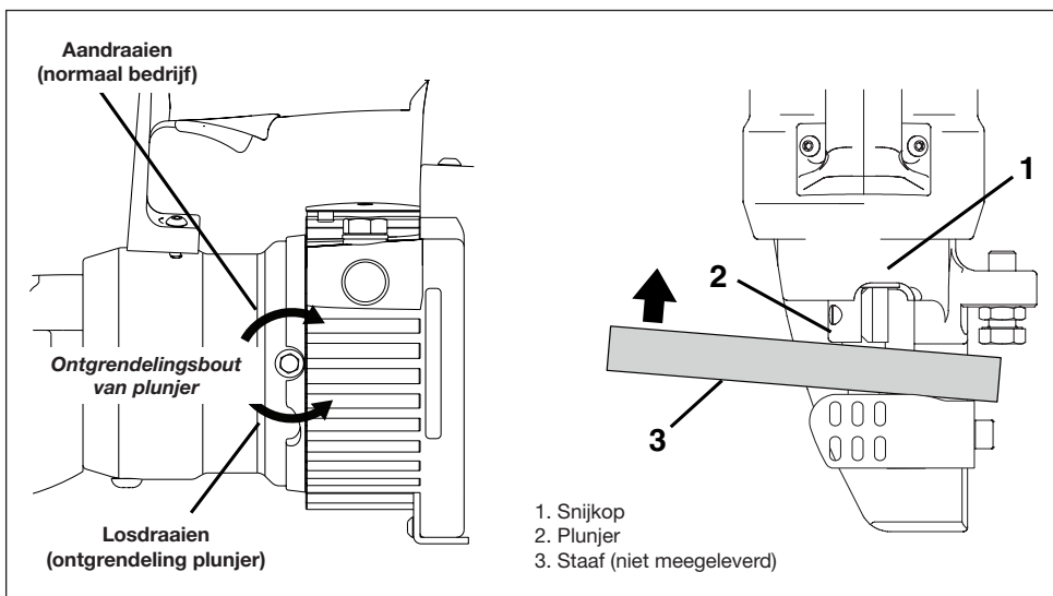
Figuur 11. Plunjer handmatig intrekken
