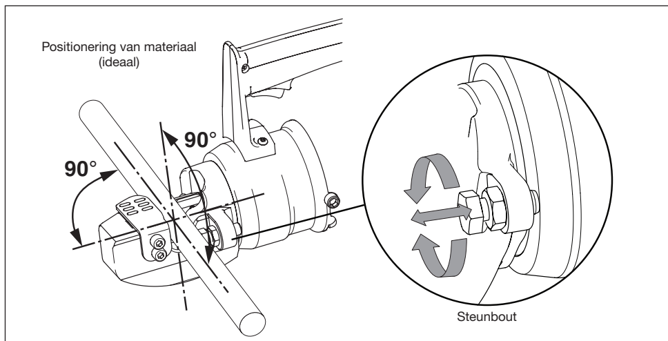
Figuur 6. Materiaal binnen in de snijkop plaatsen
