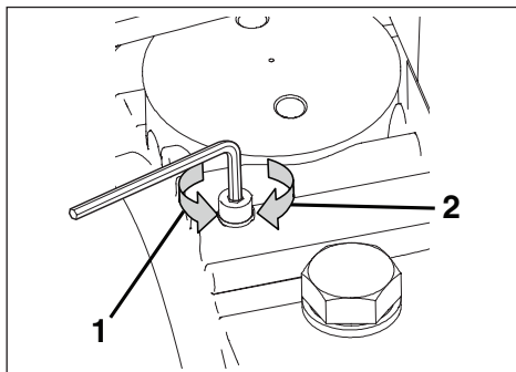
Figuur 8B. Ontluchtingsschroef losdraaien (1) en vastdraaien (2)
