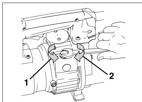
Figuur 8C. Dop van oliereservoir losdraaien (1) en vastdraaien (2)
