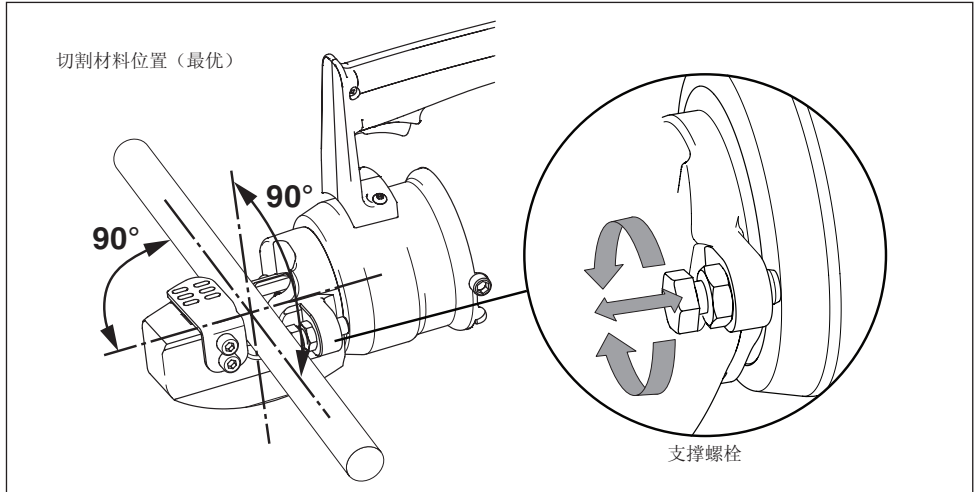
图 6，在切割头中放置切割材料
