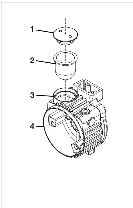
图 8E, 螺钉 (1)、隔膜盖 (1), 隔膜 (2), 隔膜口 (3) 和油箱 (4)
