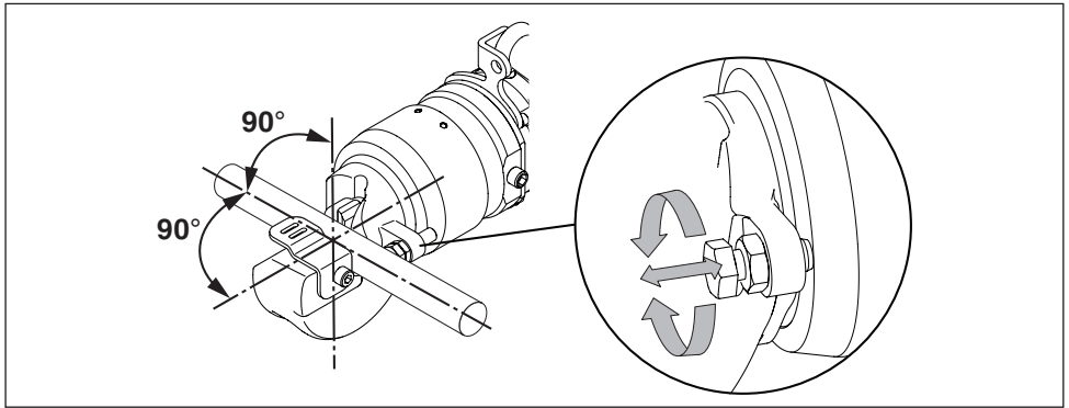
그림 12. 커팅 헤드 내부의 재료 포지셔닝
