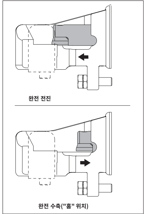
그림 8, 피스톤 위치 (평면도)
