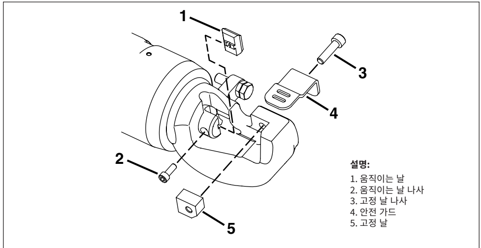
그림 16, 고정날과 움직이는 날의 교체
