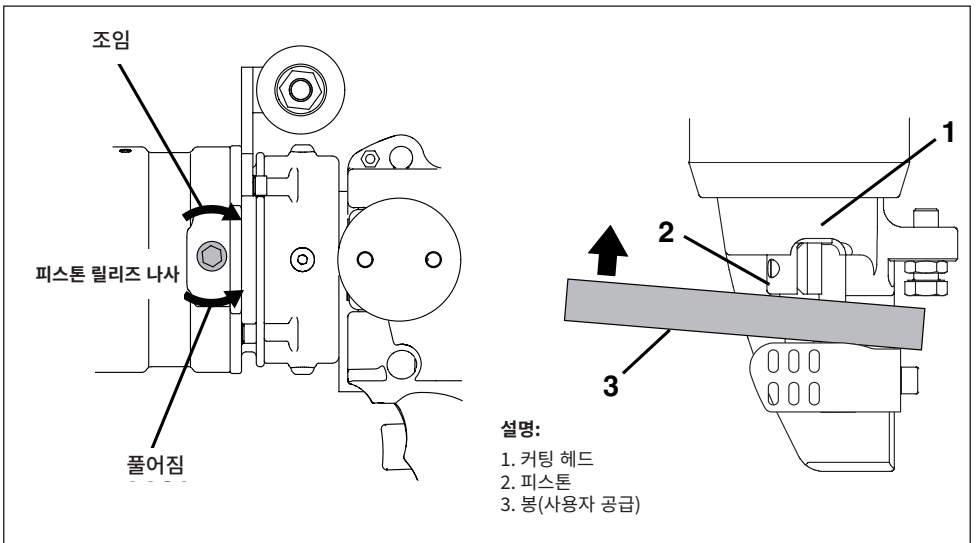
그림 17, 피스톤 수동 후진 절차
