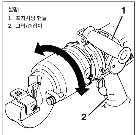
그림 5, 커팅 헤드 회전
