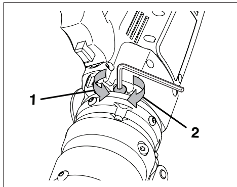
그림 15B, 오일 저장소 캡 - 플림(1) 및 조임(2)
