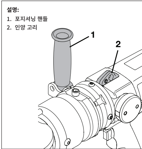
그림 11, 포지셔닝 핸들 및 리프팅 아이
