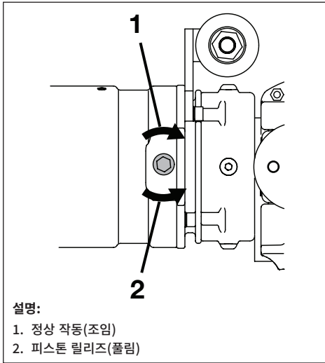
그림 9, 피스톤 릴리즈 나사
