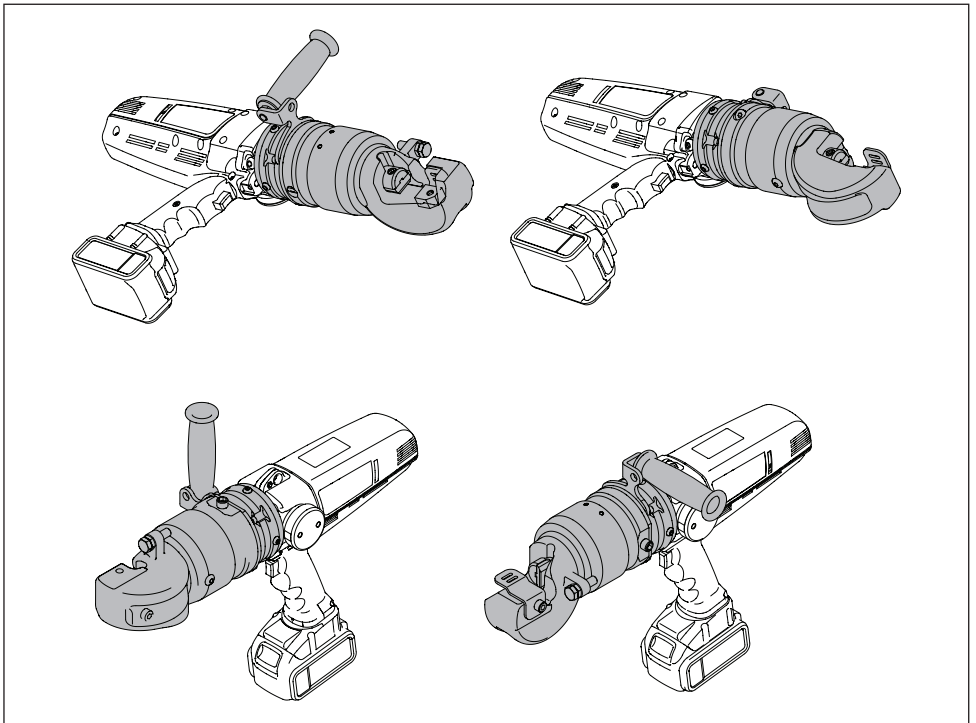
그림 6, 커팅 헤드 위치
