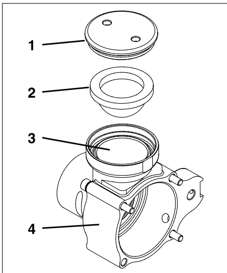
그림 15D, 다이어프램 커버(1), 다이어프램(2), 다이어프램 입구(3) 오일 저장소(4)
