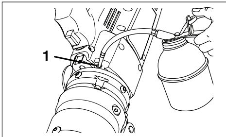
그림 15C, 저장소 보충 구멍에 오일 추가(1)
