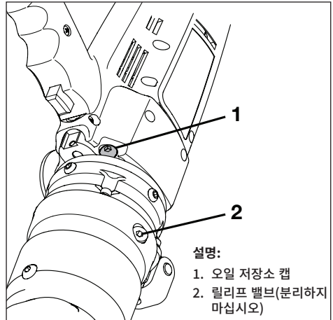
그림 14, 오일 배출/보충 캡(뒤집힌 위치에 있는 절단기)
