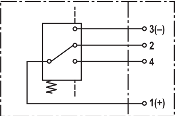
WE-1SP-M12x1 Esquema del circuito con elemento de conmutación montado en filtro sin presión
