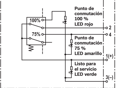
WE-2SP-M12x1 Esquema del circuito con elemento de conmutación montado en filtro sin presión
