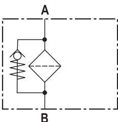
Filtro de retorno para montaje con bypass
