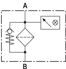
Filtro de retorno para montaje con bypass e indicador mecánico
