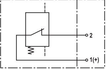
WE-1SP-EN175301-803 Esquema del circuito con elemento de conmutación montado en filtro sin presión
