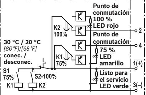
WE-2SPSU-M12x1 Elemento de conmutación montado en filtro sin presión a una temperatura > 30 °C [86 °F]
