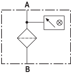
Filtro de retorno para montaje sin bypass y con indicador mecánico
